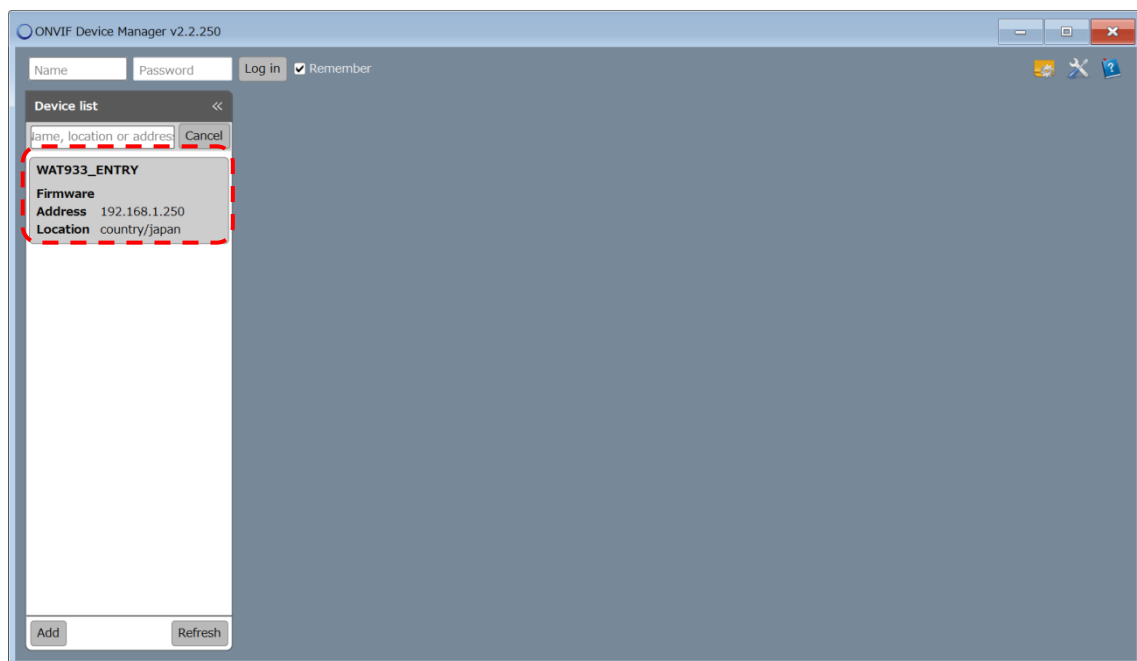
図 49. ODM 画面
