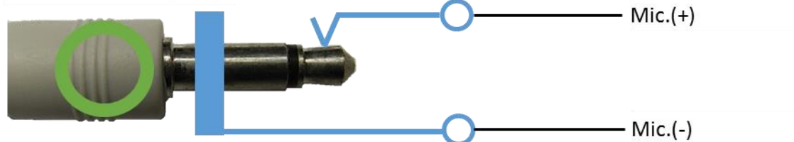
図 7. 正しい接続例
