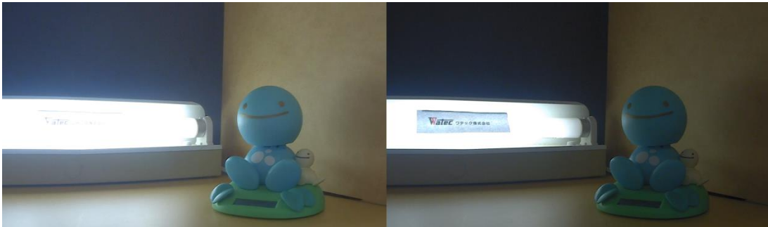
図 26. (左)Anti Saturation:OFF、(右)Anti Saturation:ON
