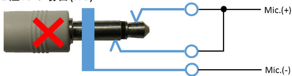
図 8. 間違った接続例
