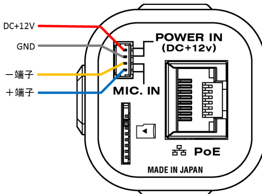
図 9. 4P ケーブルの配線図
