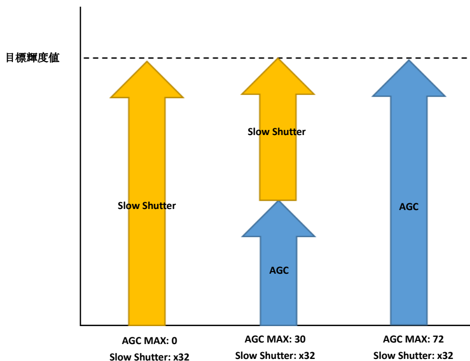
図 27. AGC と Slow Shutter の関係性
