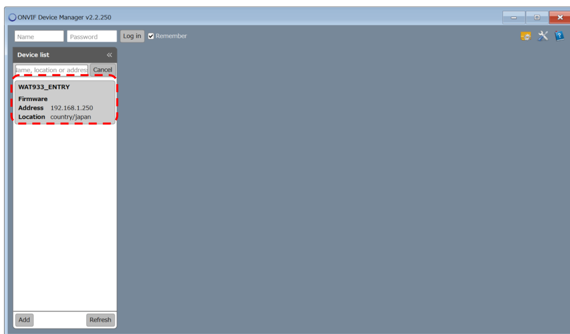
図 48. ODM 画面
