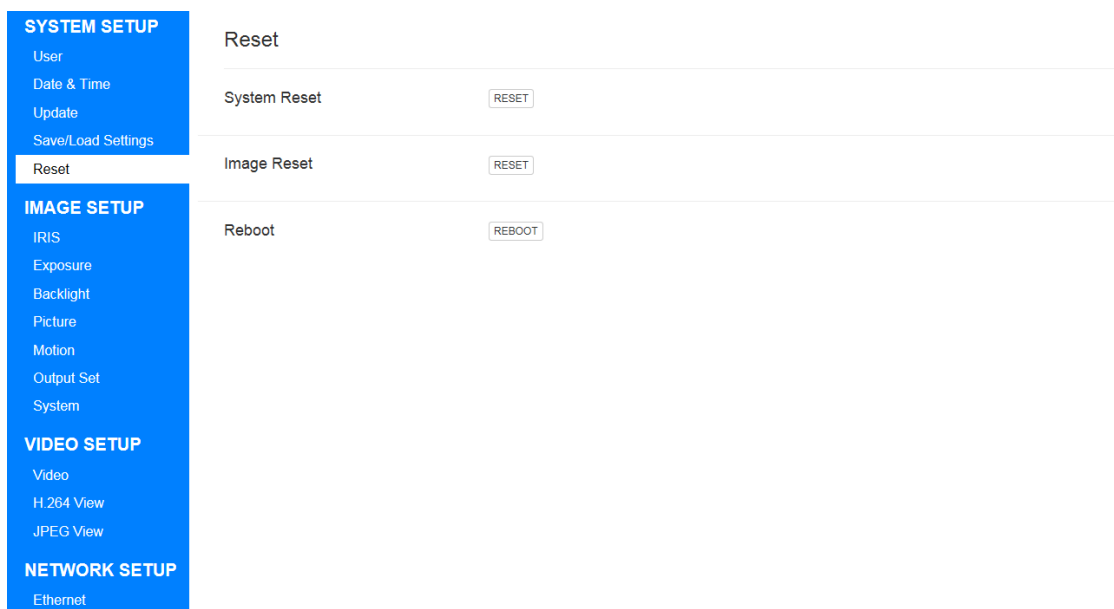
図 23. Reset 画面
