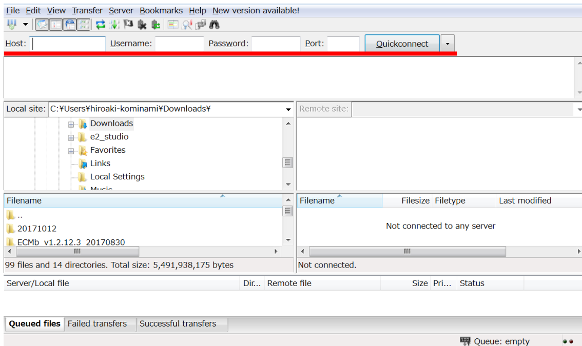
図 51. FileZilla 画面
